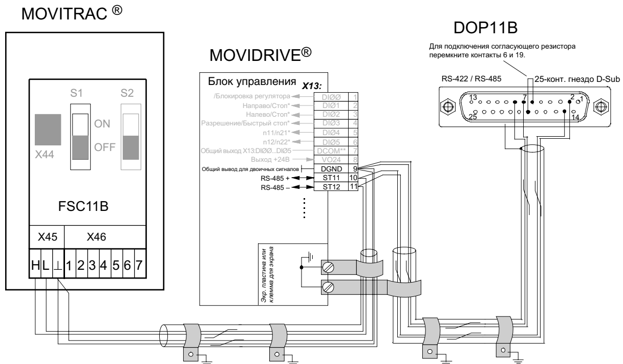
Рис. 11. Назначение выводов панели DOP11B
