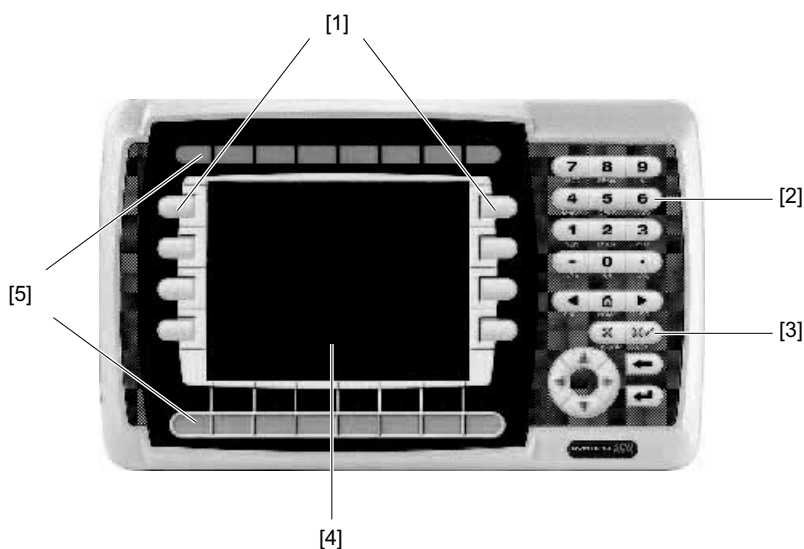
Рис. 5. DOP11B-40
