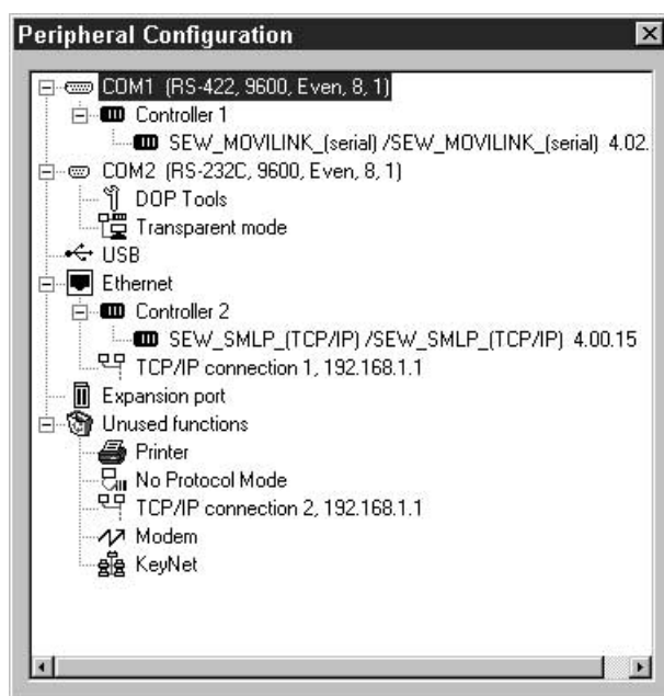
Рис. 25. Настройка параметров обмена данными
