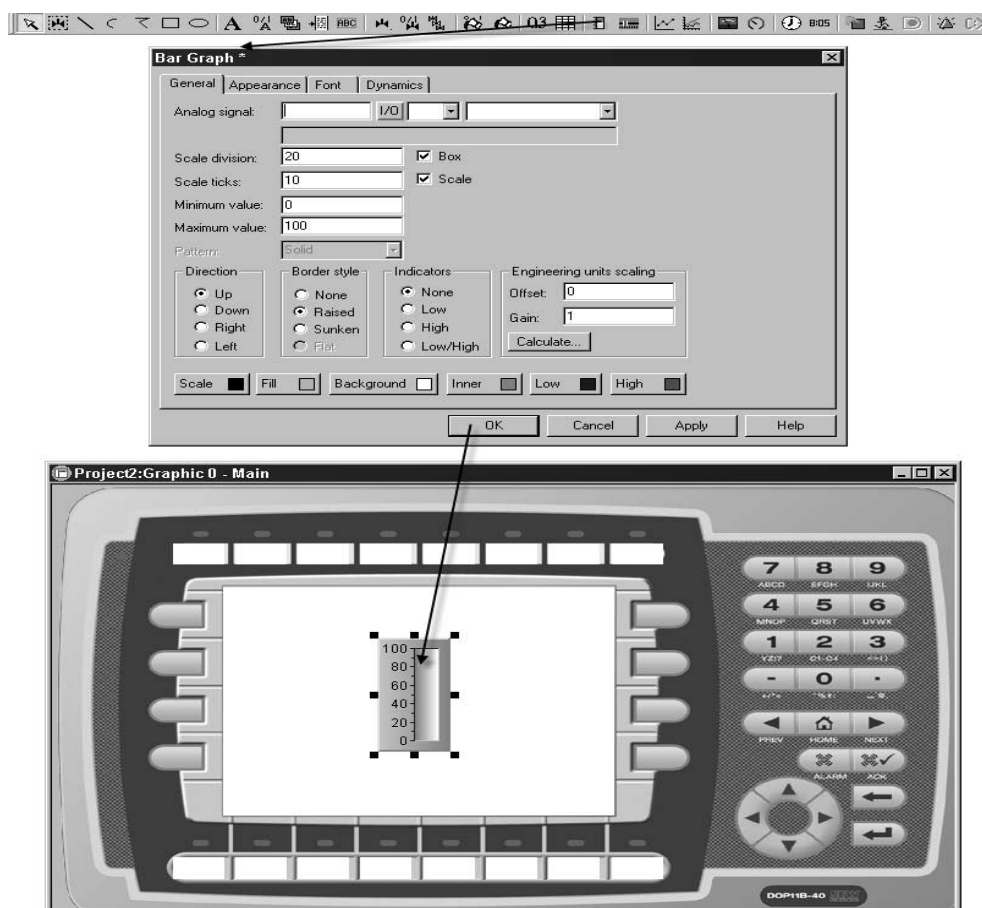
Рис. 39. Программирование блоков
