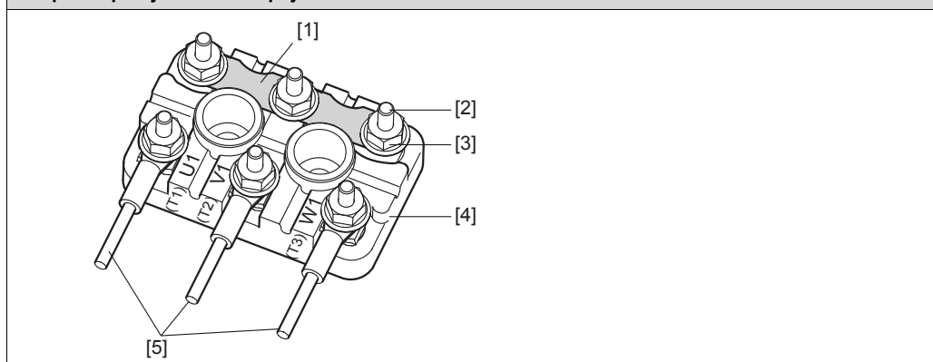
Raspored priključaka kod spoja u \Delta
