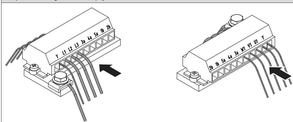
Raspored steznog mosta za vezu u △
