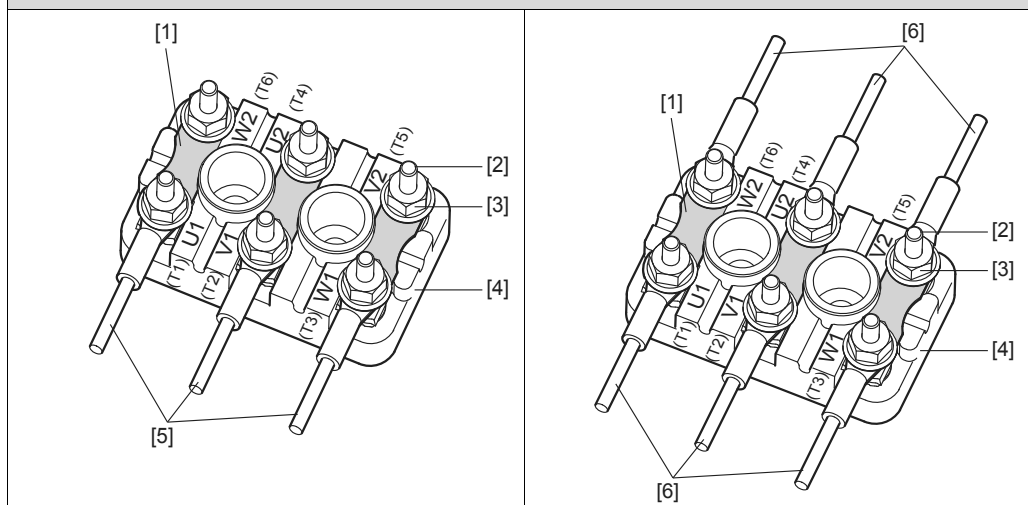
Raspored priključaka kod spoja u \Delta
