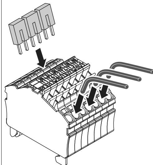
Raspored steznog mosta za vezu u \Delta
