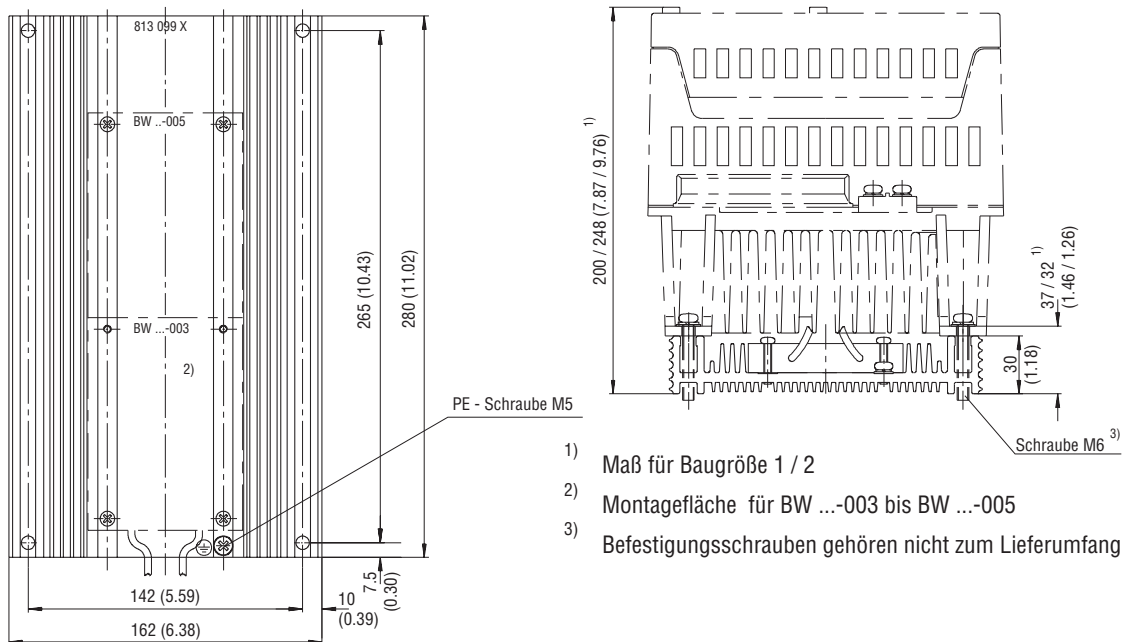
Bild 1: Montagekühlkörper FKB01 für Bremswiderstände, Maße in mm (in)
