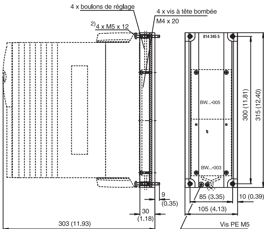
Fig. 1 : Cotes en mm (in) du radiateur DKB11A
