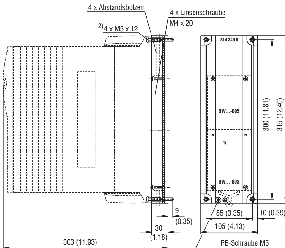
Bild 1: DKB11A Montagekühlkörper für Bremswiderstände, Maße in mm (in)
